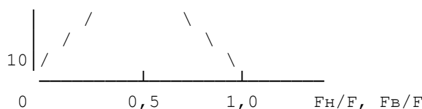
График для определения коэффициента В при расчете коэффициента k4
